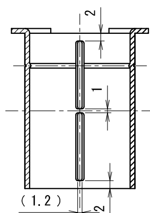
B-B断面図
