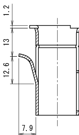
A-A断面図
