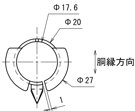
閉じた状態
